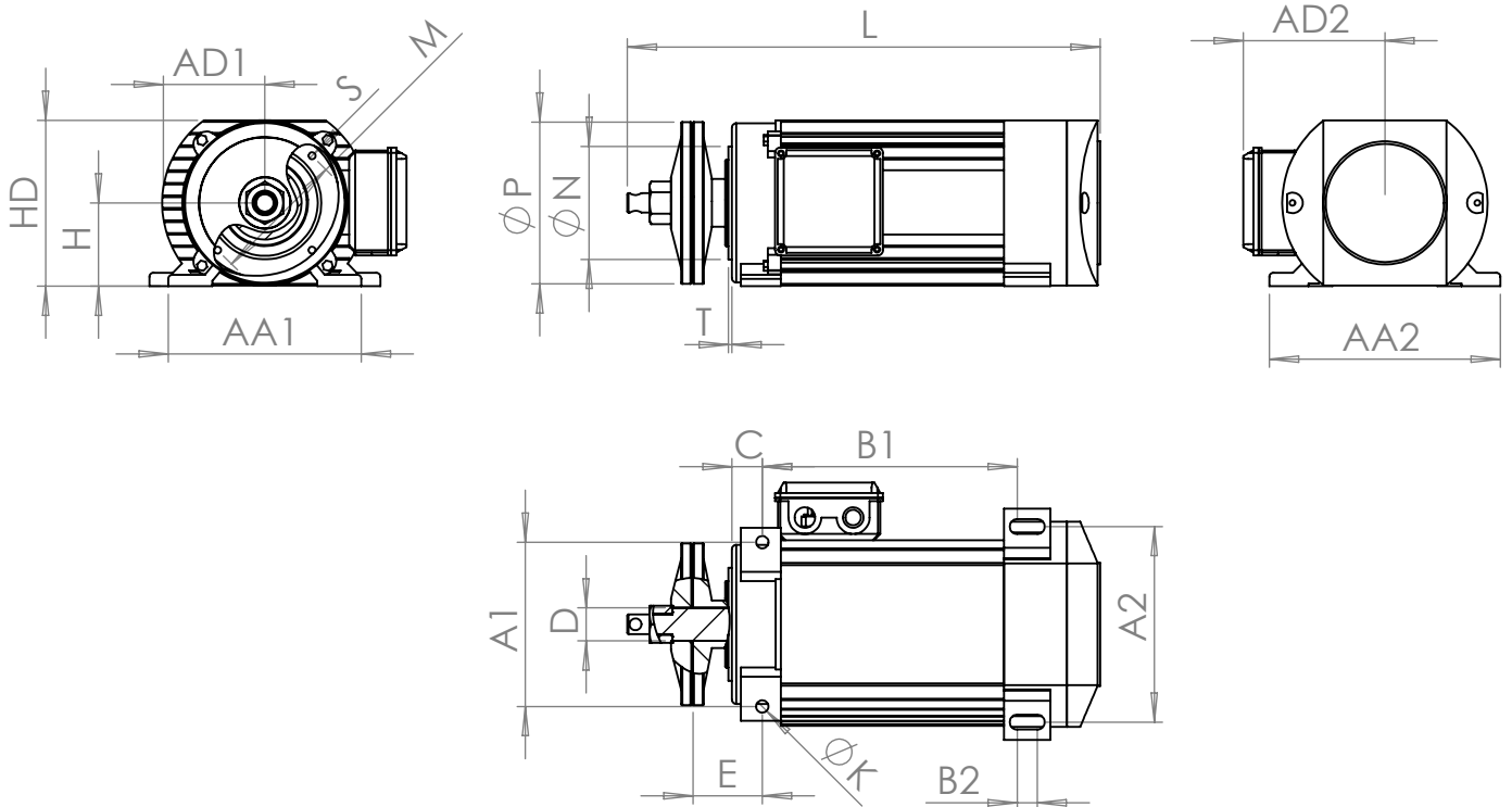
Maßblatt Flachmotor mit Klemmflansch -Serie KSE / KSD- [mm] dimensions flat motor with clamping flange -Serie KSE / KSD [mm]
